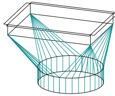
TRANSICIÓN EXCÉNTRICA
