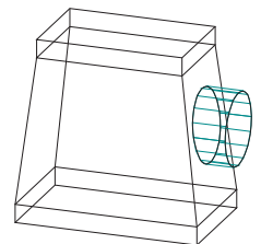
CUADRADO CON INJERTO REDONDO
