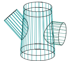
CRUZ / INJERTO 45 Y 90°
